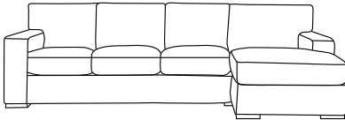
3 SEATER + CHAISE 326w 157d 87h 279w 150d 87h
