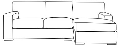
2.5 SEATER + CHAISE 285w 157d 87h 254w 150d 87h
